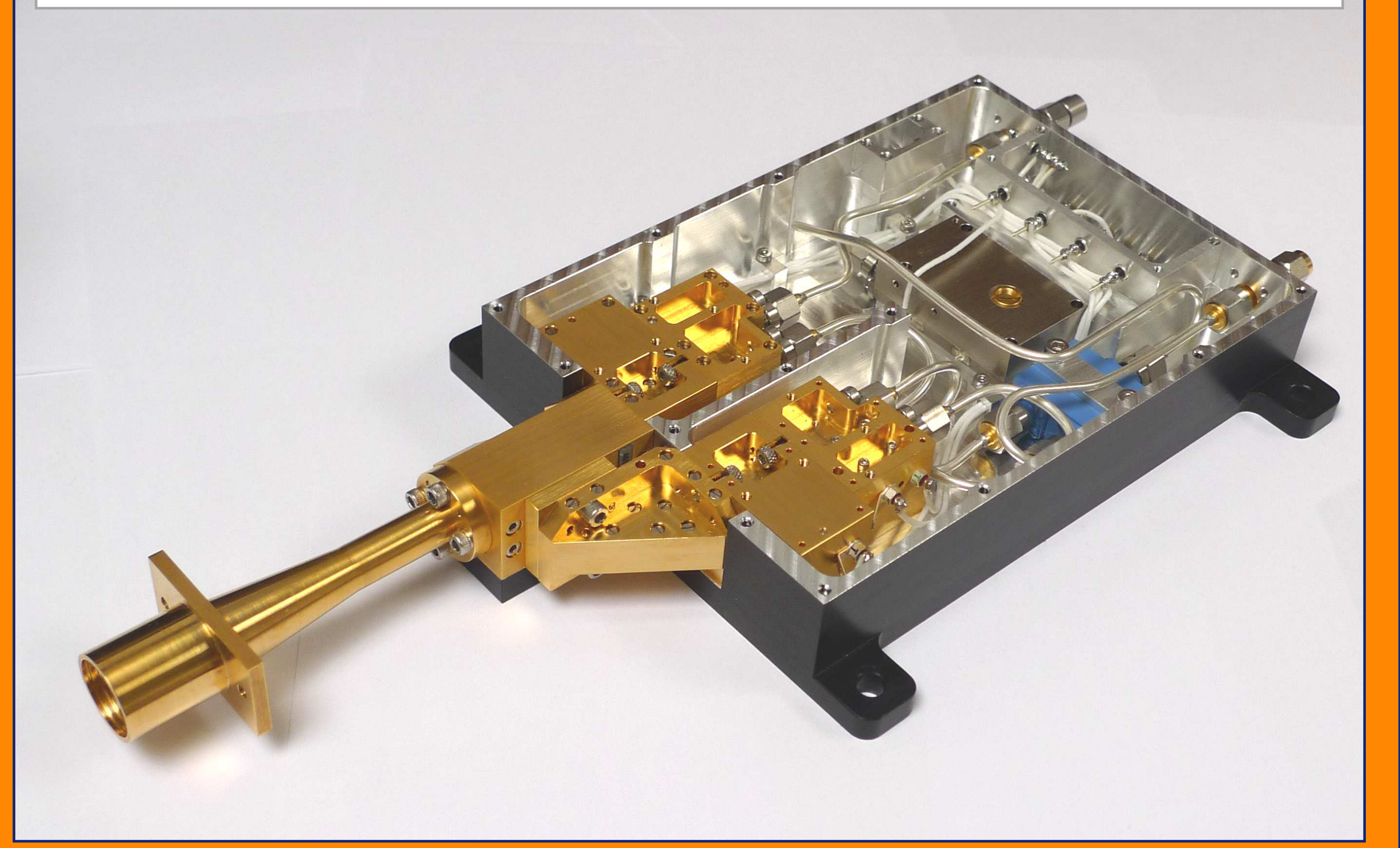
89 GHz MHS-II, China, FY-3
