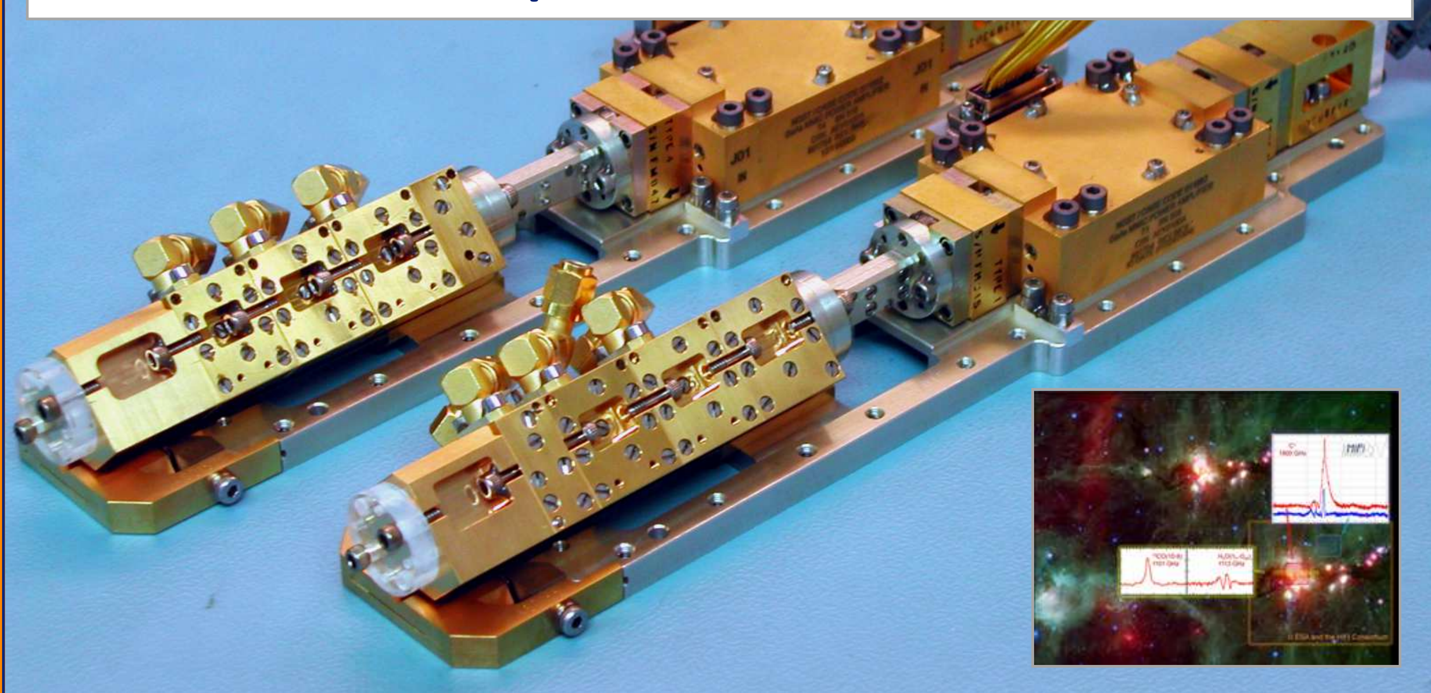
Herschel/HIFI 1100 GHz LO
