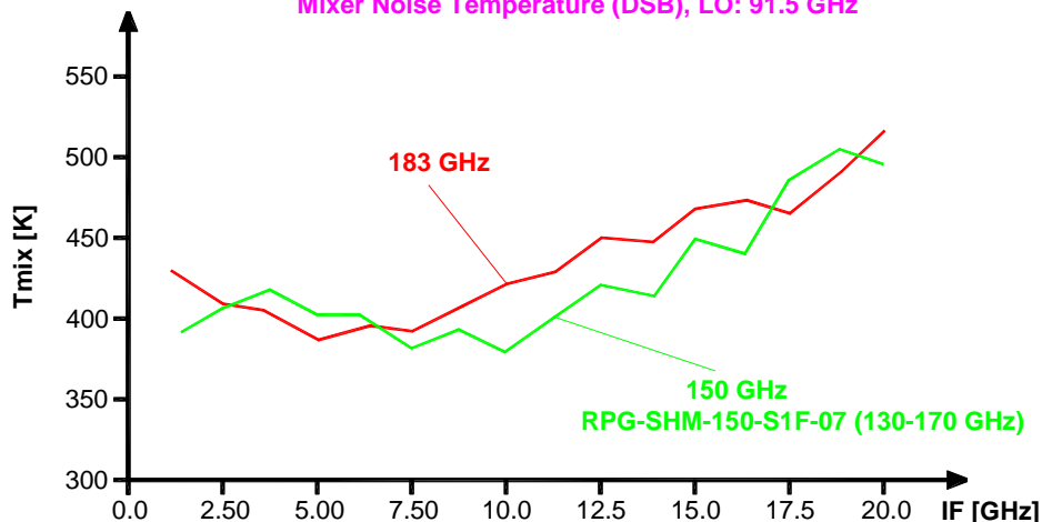
183 GHz SHM RPG-SHM-183-S1F-19 (167-200 GHz)
